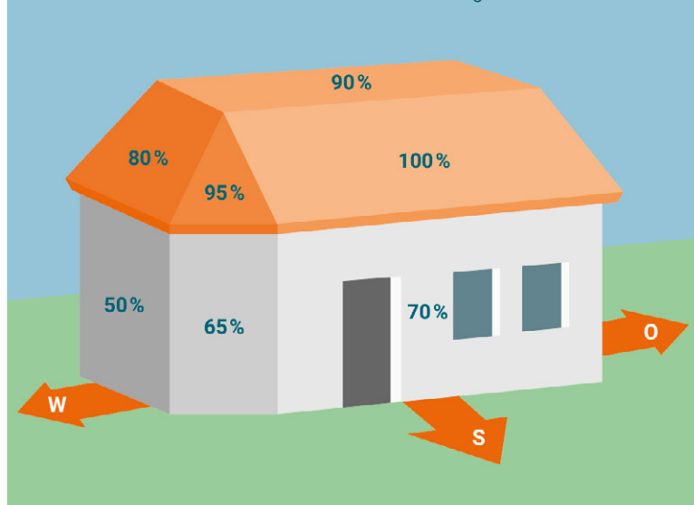
Prozentualer Ertrag bei unterschiedlichen Ausrichtungen und Neigungen des Dachs im Verhältnis zur idealen Südausrichtung
