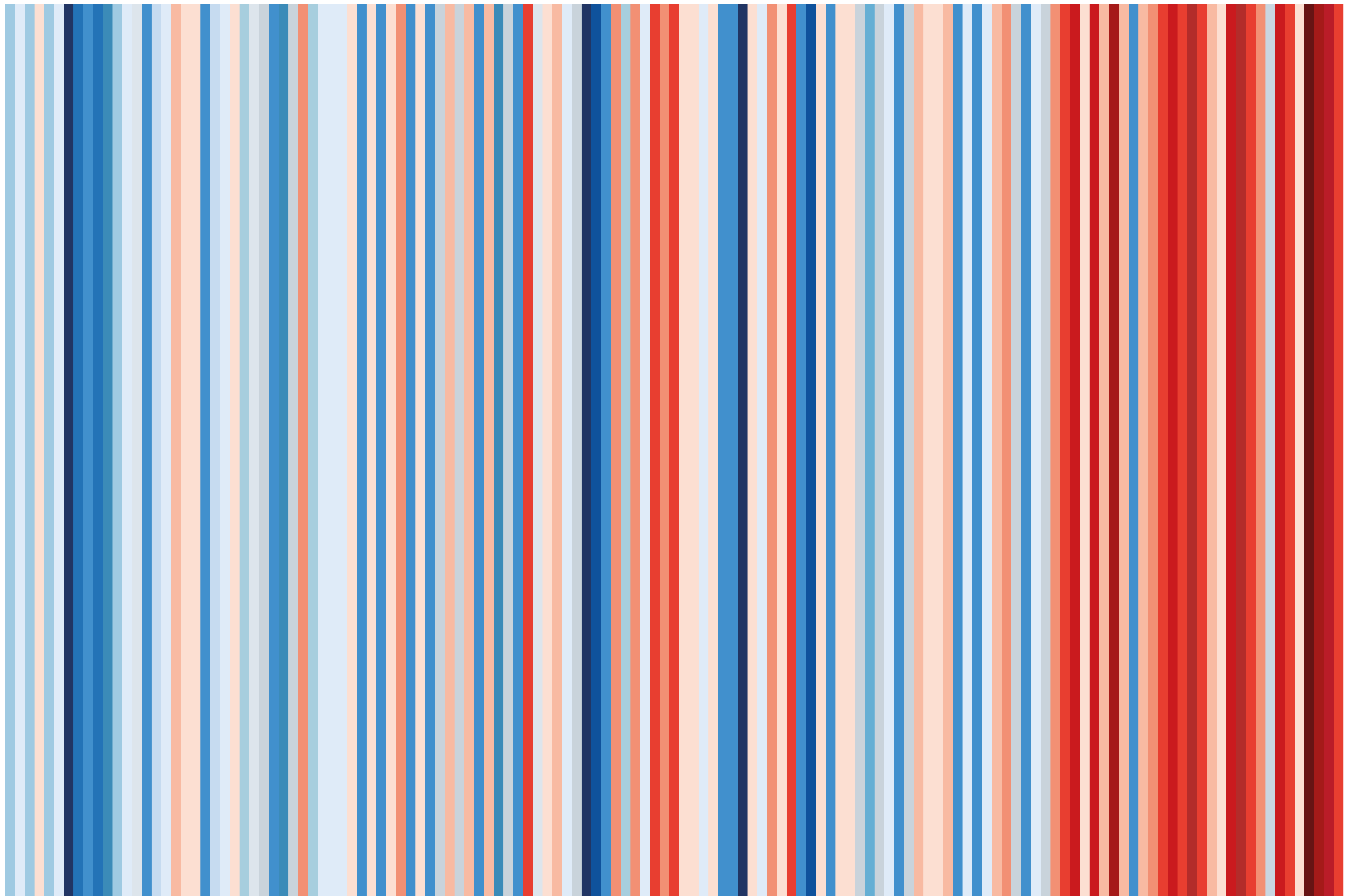
Jahresmitteltemperatur in Baden-Württemberg seit Beginn der Wetteraufzeichnungen 1881 bis 2017
